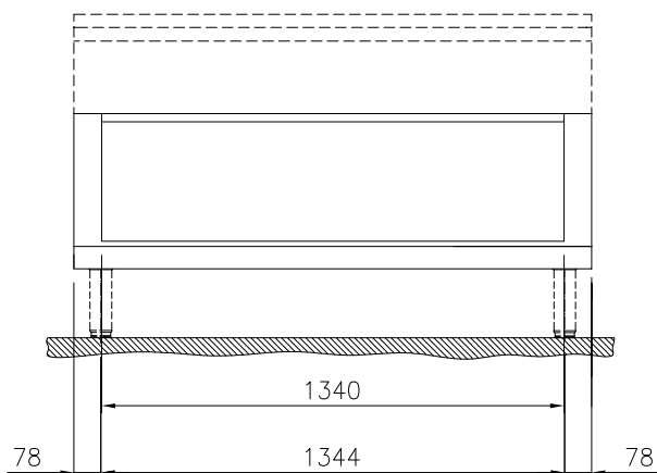
Fronte
